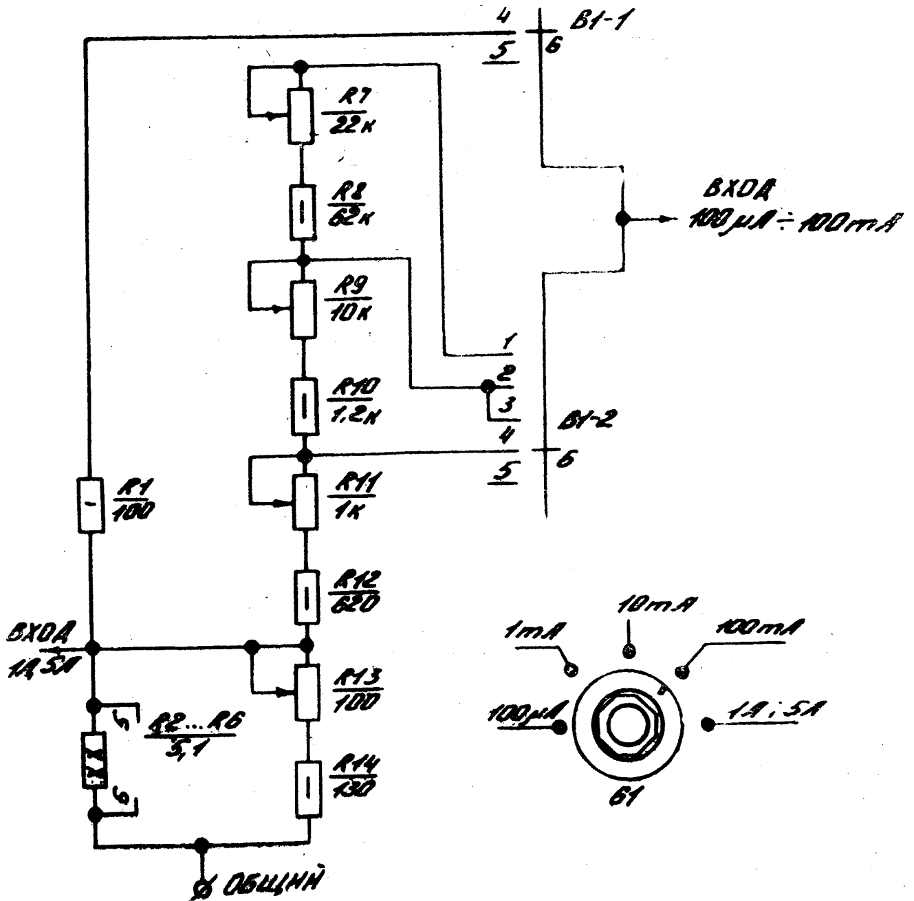
Рис. 1. Схема устройства для регулировки силы постоянного тока
